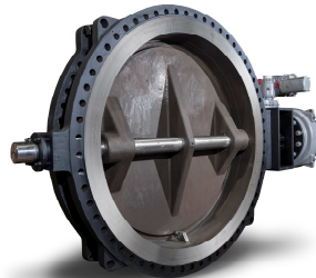
72 CI150 Lug CF8M Upstream View
