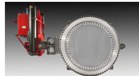
84 CI300 Lug 347sst x Inconel Flare Gas Service
